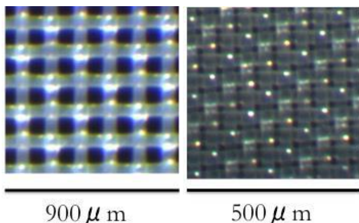
Figur 30. Nærbilleder af de to anvendte Hydrotech polyester filterduge. Til venstre ses 100 µm filterdugen og til højre ses 25 µm filterdugen. Under hvert billede er størrelsen af feltet angivet.
