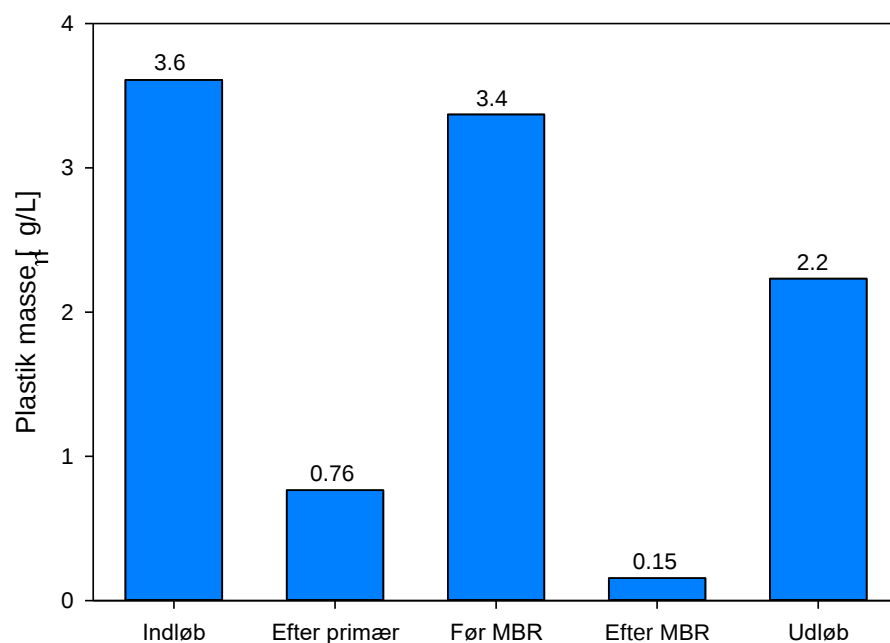
Figur 14. Koncentration af mikroplast målt som plast masse per liter vand på Renseanlæg A.
